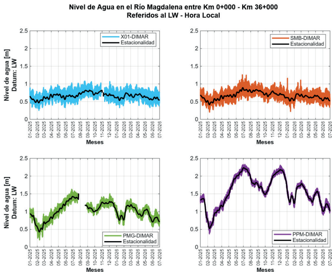
Figura 40. Serie temporal comportamiento niveles de agua y estacionalidad en el Río Magdalena (km 0 al km 36).
