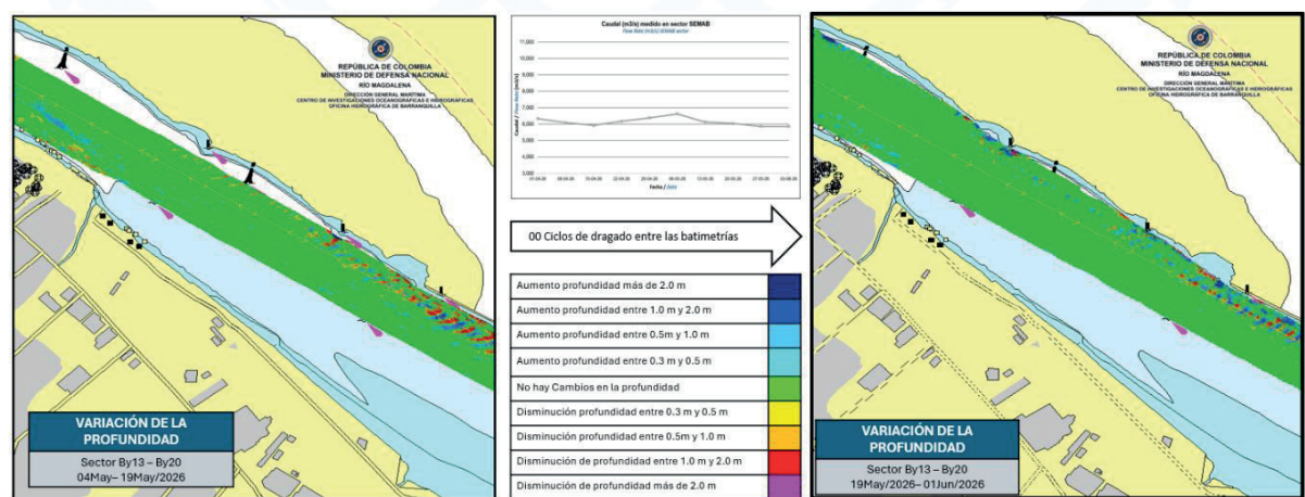
Figura 21. Diferencia de superficie entre el 19 de mayo y 01 de junio del 2026.
