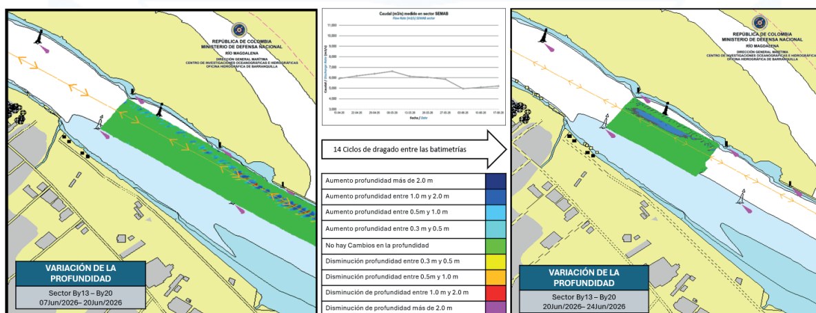
Figura 24. Diferencia de superficie entre el 20 y 24 de junio del 2026.
