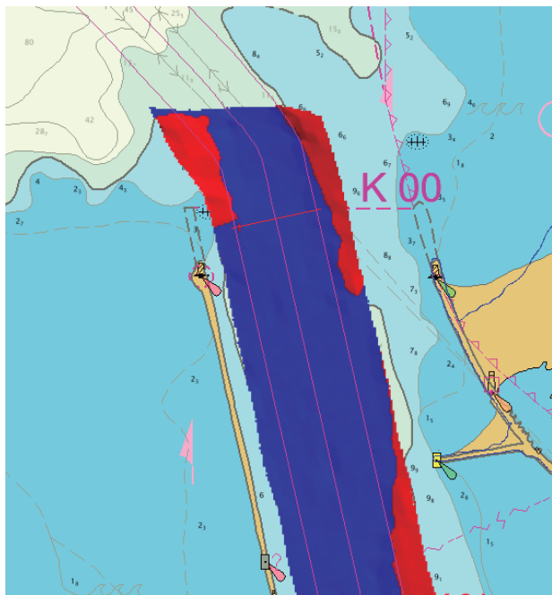
Figura 4. Evolución Condiciones Canal Navegable, sector bocas de cenizas. Levantamientos batimétricos durante el mes de febrero del 2022
