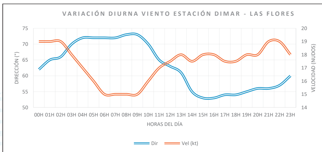
Figura 11. Serie horaria variación diurna viento en el sector Las Flores (febrero 2022 – Promedio x hora).
