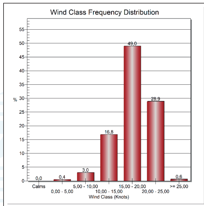
Figura 15. Distribución de frecuencia viento (nudos) en el sector Las Flores (febrero 2022).
