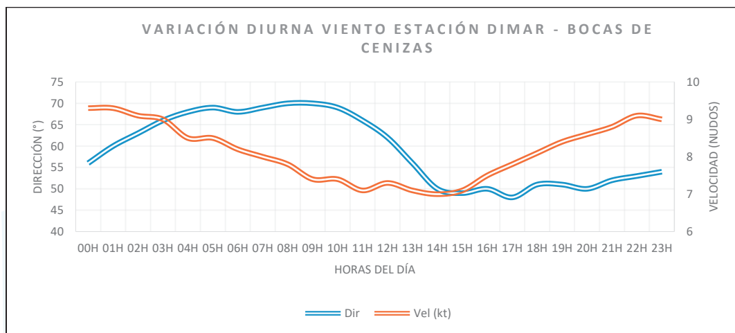
Figura 13. Serie horaria variación diurna viento en Bocas de Cenizas (febrero 2022 - Promedio x hora).
