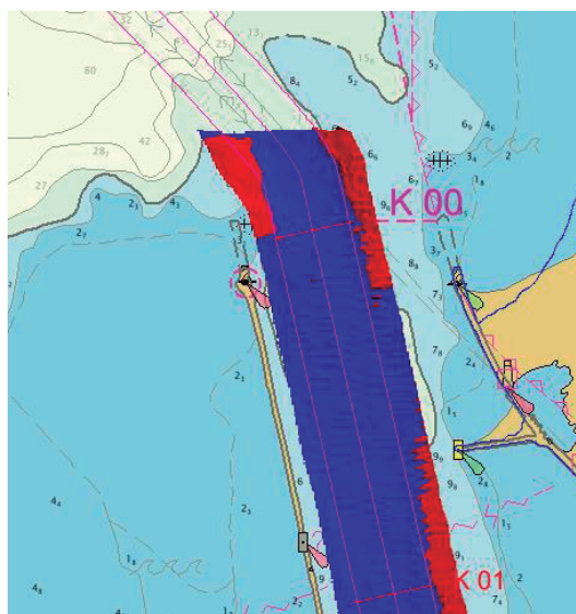
Figura 3. Condiciones Canal Navegable, sector bocas de cenizas. Levantamientos batimétricos durante el mes de febrero de 2022, profundidad de referencia 11.5 m. Calado Operativo del puerto 10 m.
