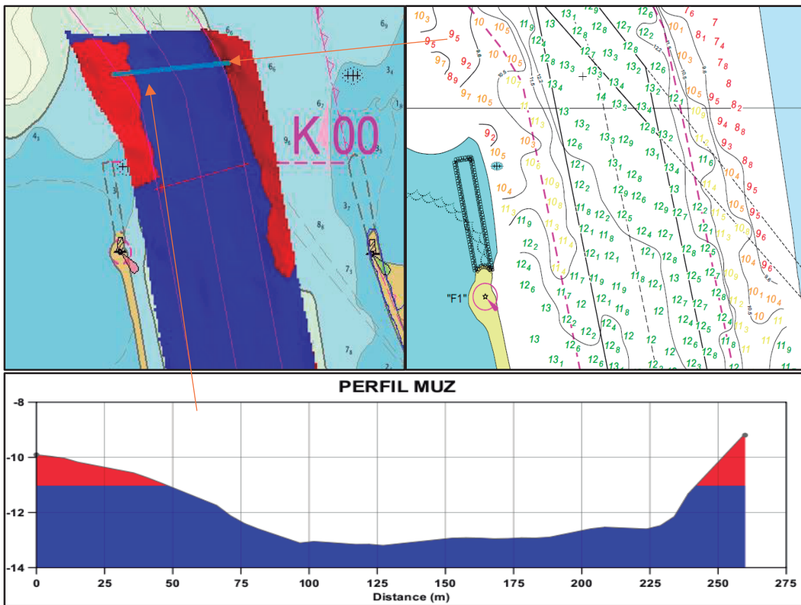
Figura 5. Perfil batimétrico, sector bocas de cenizas. Levantamiento batimétrico del 28 de febrero de 2022, profundidad de referencia 11.5 m. Calado Operativo del puerto 10 m
