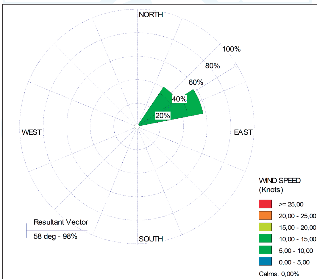
Figura 14. Rosa general distribución del viento en el sector Bocas de Cenizas (febrero 2022 – Serie horaria).
