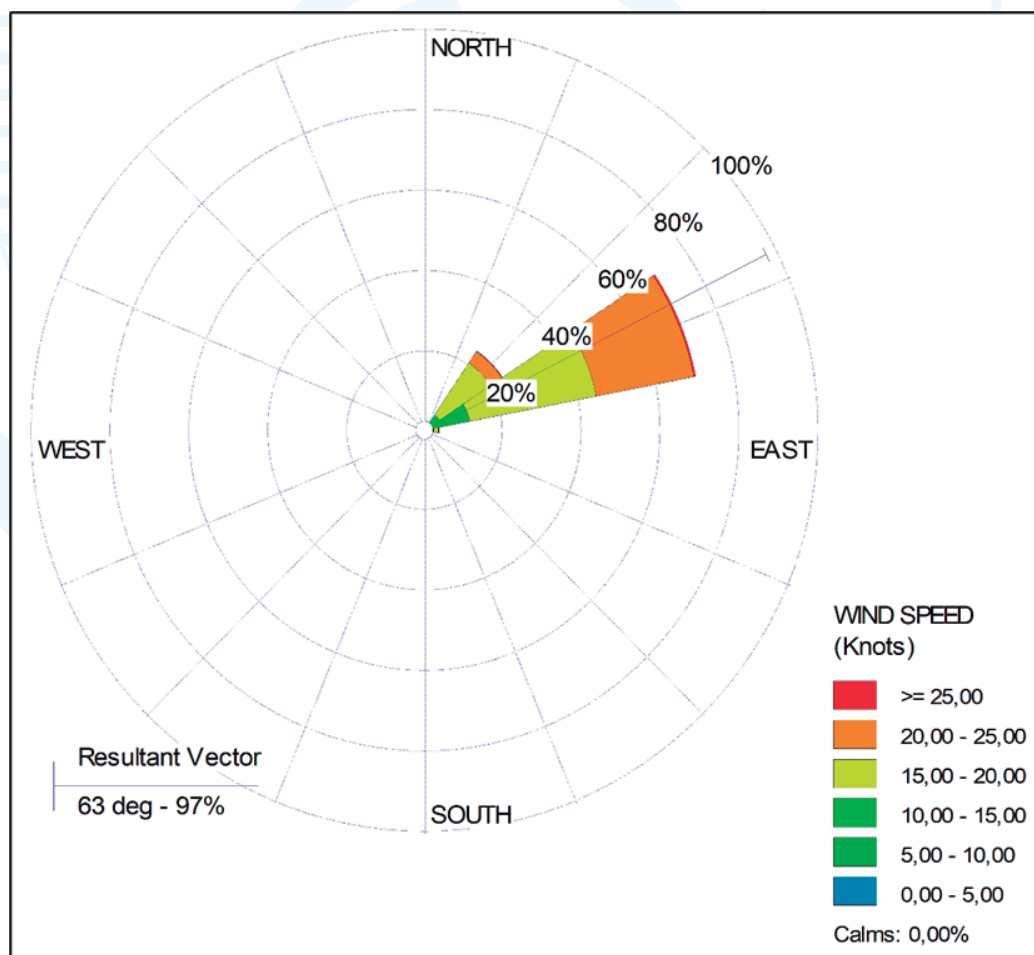
Figura 12. Rosa general distribución del viento en el sector Las Flores (febrero 2022 – Serie horaria).
