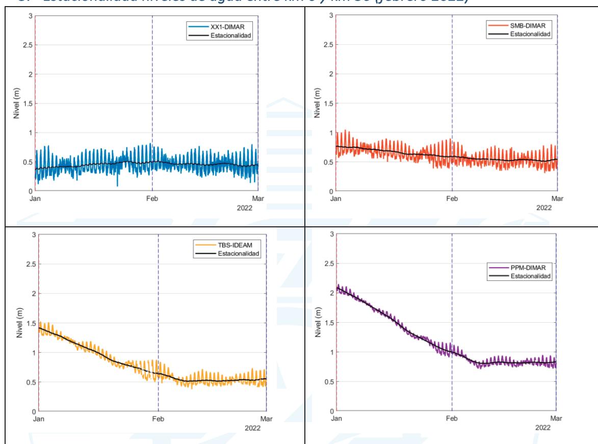
Figura 10. Serie temporal comportamiento niveles de agua en el Río Magdalena (km 0 al km 36).
