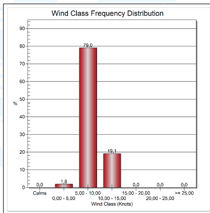
Figura 16. Distribución de frecuencia viento (nudos) en el sector Bocas de Cenizas (febrero 2022).
