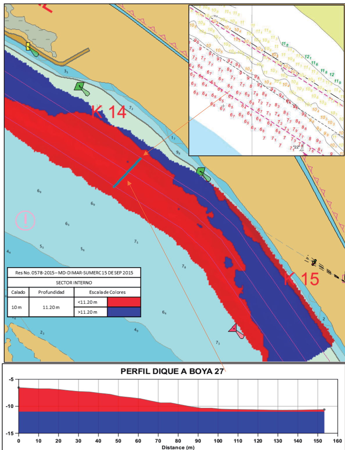
Figura 7. Dique Direccional a Boya 27 (km 13 a km 16) – Perfil batimétrico área menos profunda. Levantamiento batimétrico del 05 de febrero de 2022.
