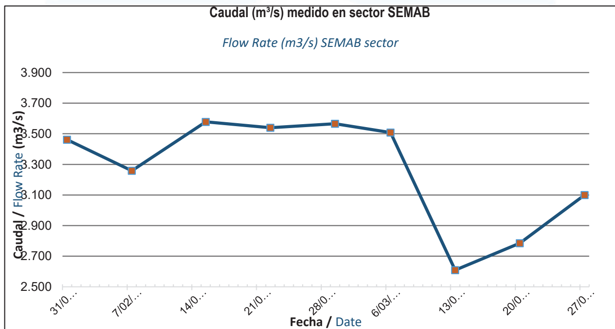
Figura 26. Evolución comportamiento caudal sección transversal km 8+500.
