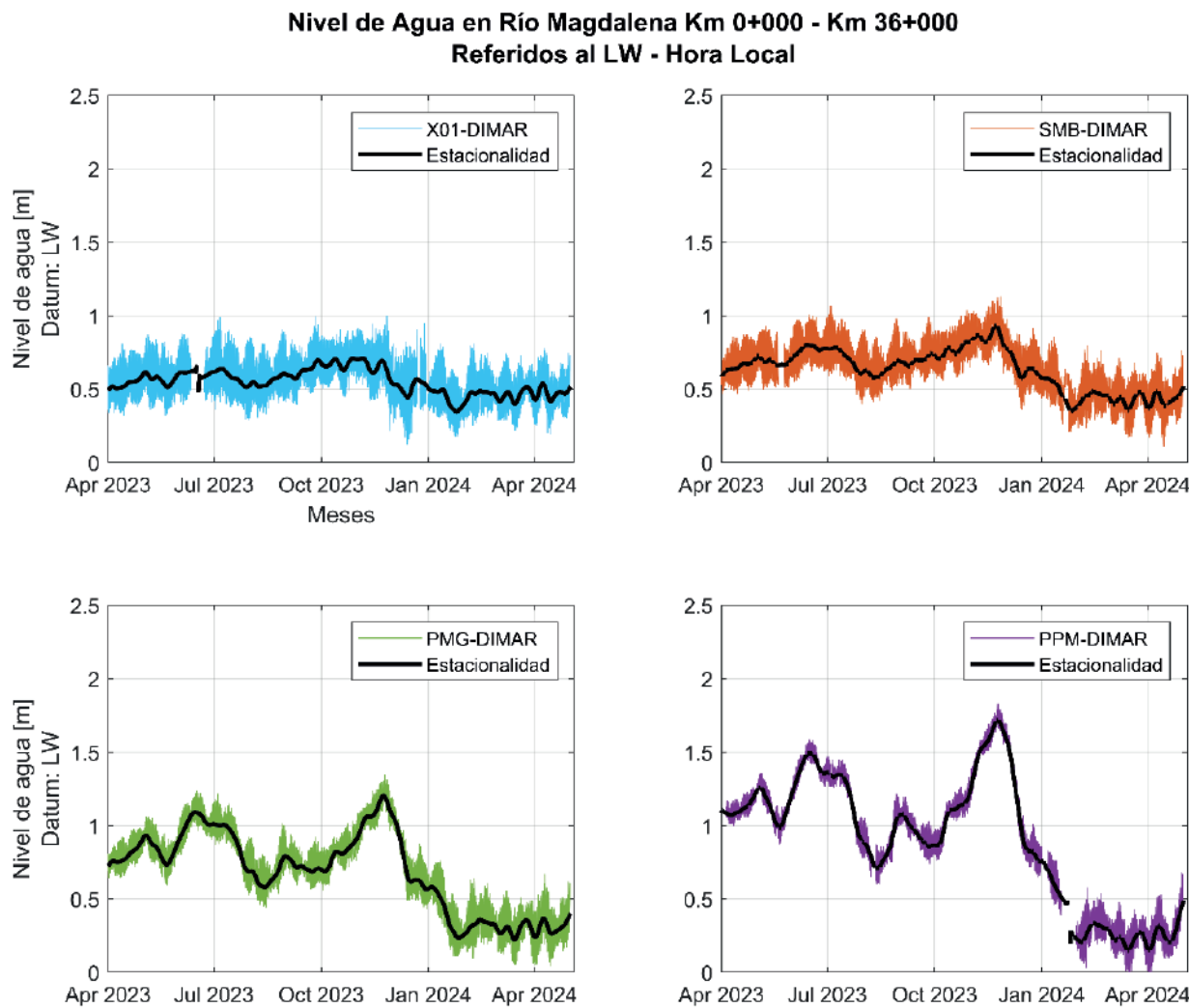
Figura 33. Serie temporal comportamiento niveles de agua y estacionalidad en el Río Magdalena (km 0 al km 36).
