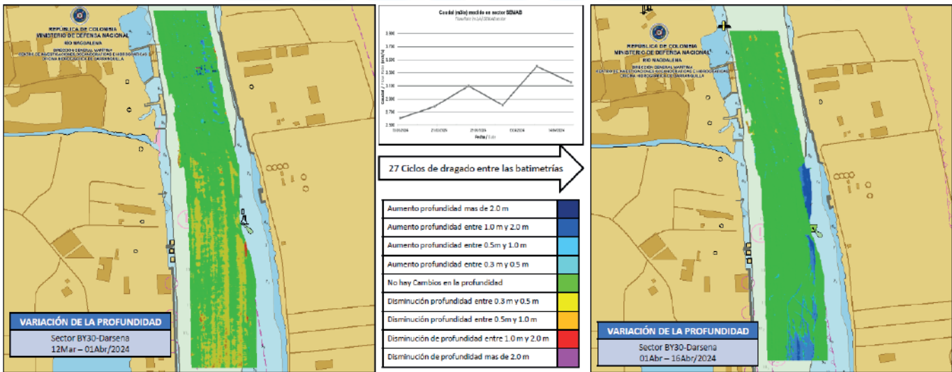
Figura 23. Diferencia de superficie entre el 01 y 16 de abril del 2024.
