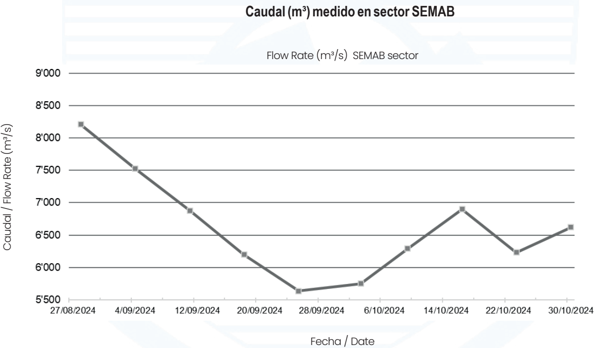
Figura 26. Evolución comportamiento caudal sección transversal km 8+500.
