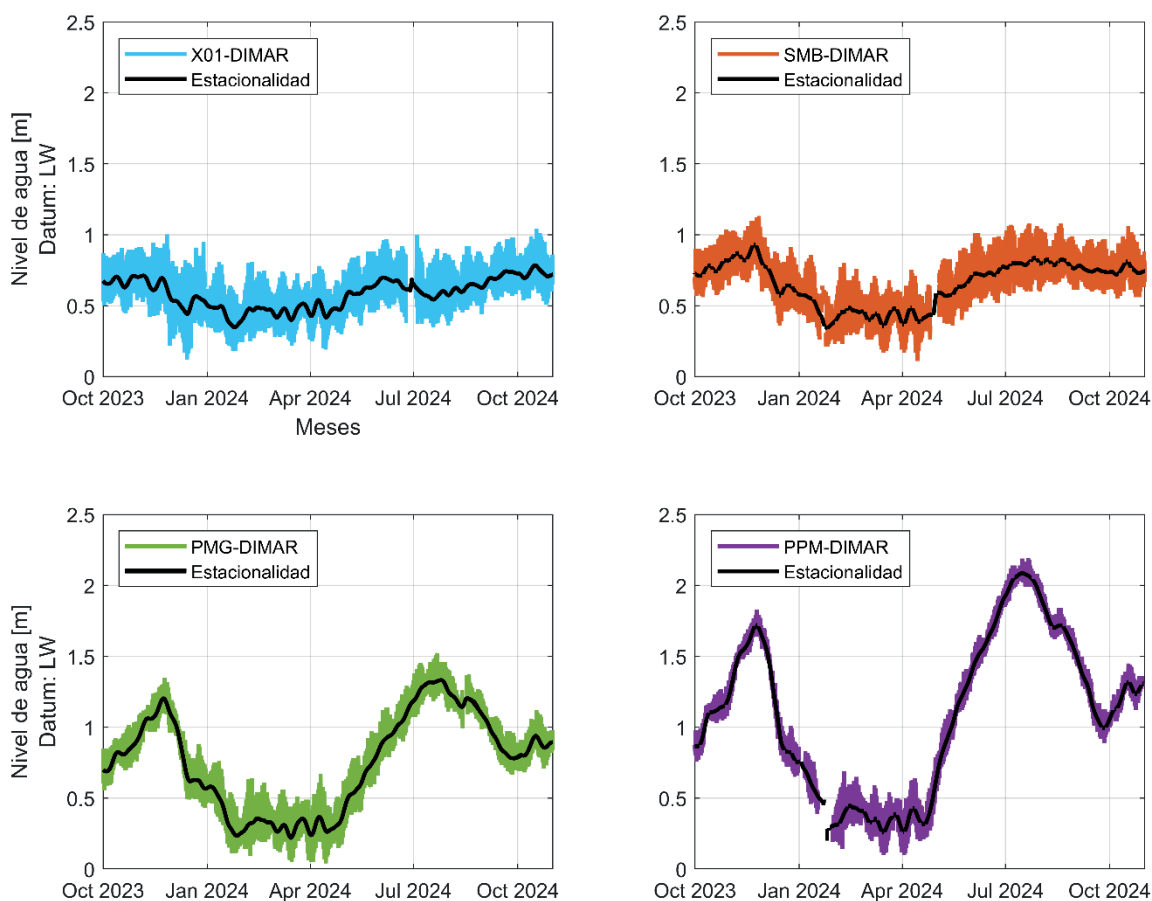
Figura 27. Serie temporal comportamiento niveles de agua y estacionalidad en el Río Magdalena (km 0 al km 36).
