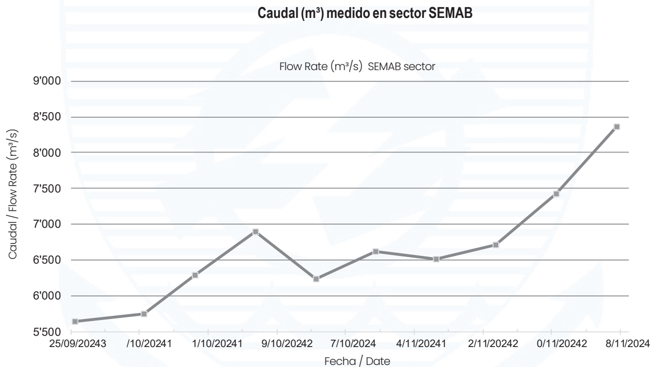
Figura 23. Evolución comportamiento caudal sección transversal km 8+500.
