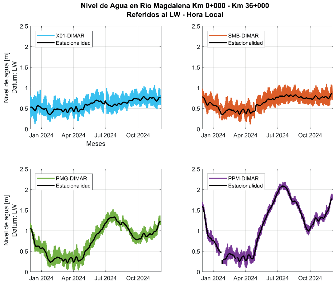
Figura 24. Serie temporal comportamiento niveles de agua y estacionalidad en el Río Magdalena (km 0 al km 36).
