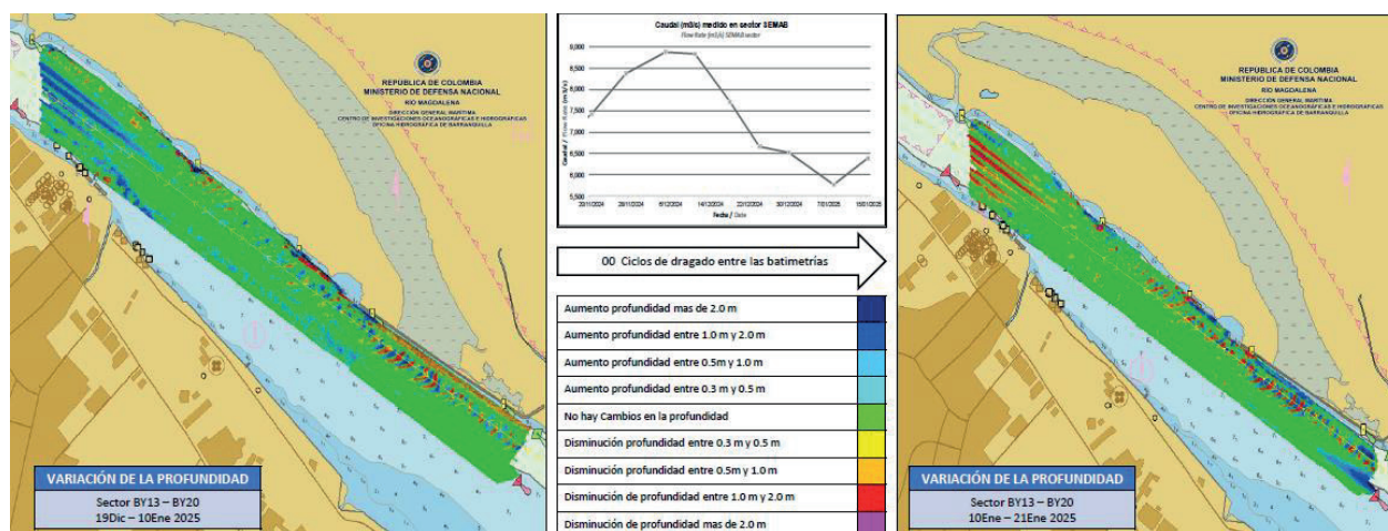
Figura 16. Diferencia de superficie entre el 10 y el 21 de enero del 2025.
