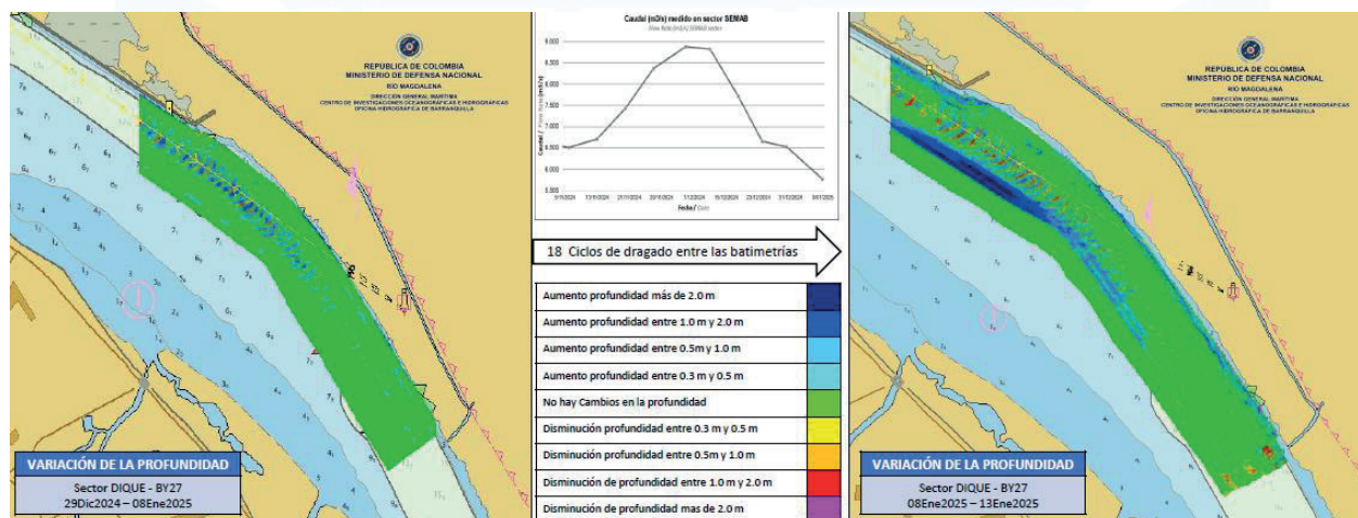
Figura 18. Diferencia de superficie entre el 08 y 13 enero del 2025.
