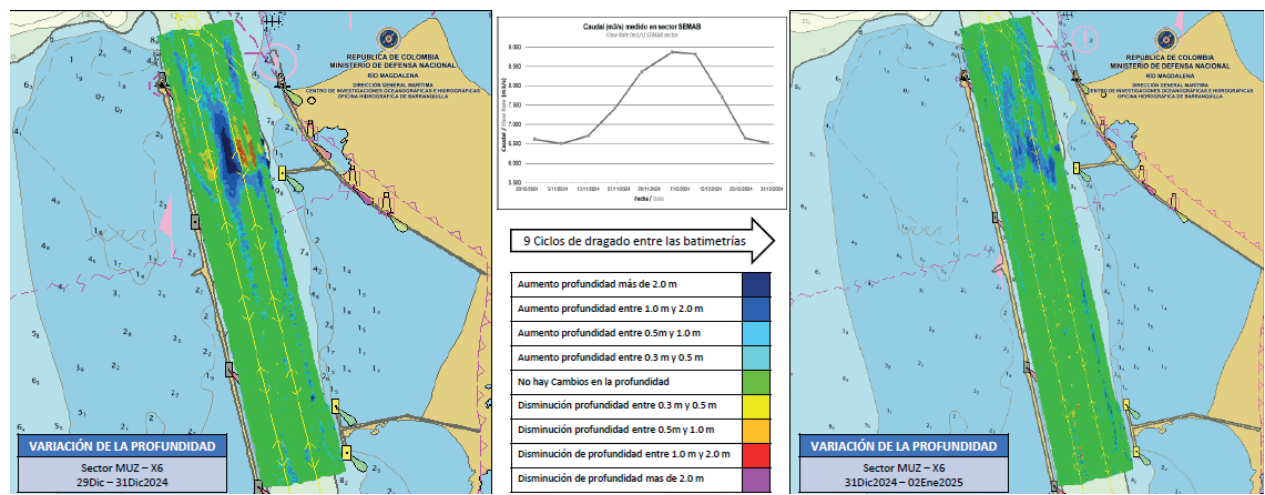
Figura 1. Diferencia de superficie entre el 31 de diciembre y el 02 de enero 2025.
