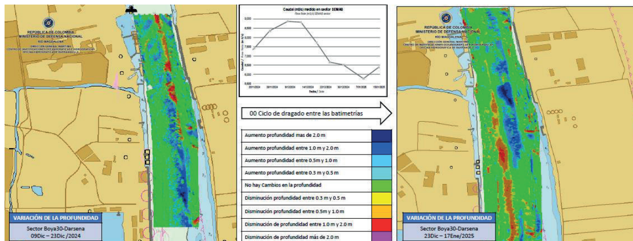
Figura 22. Diferencia de superficie entre el 23 de diciembre y el 17 de enero del 2025.
