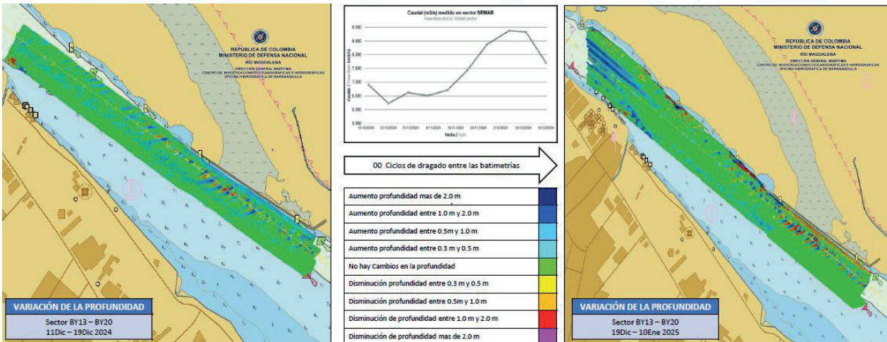
Figura 15. Diferencia de superficie entre el 19 de diciembre y el 10 de enero del 2025.
