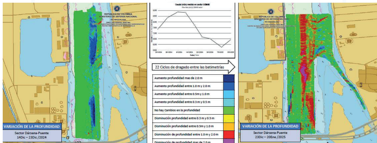
Figura 23. Diferencia de superficie entre el 23 de diciembre y el 20 de enero del 2025.
