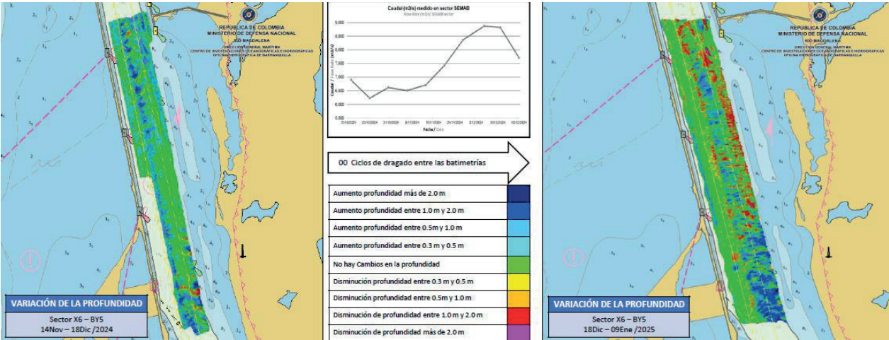
Figura 8. Diferencia de superficie entre el 18 de diciembre y el 09 de enero del 2025.
