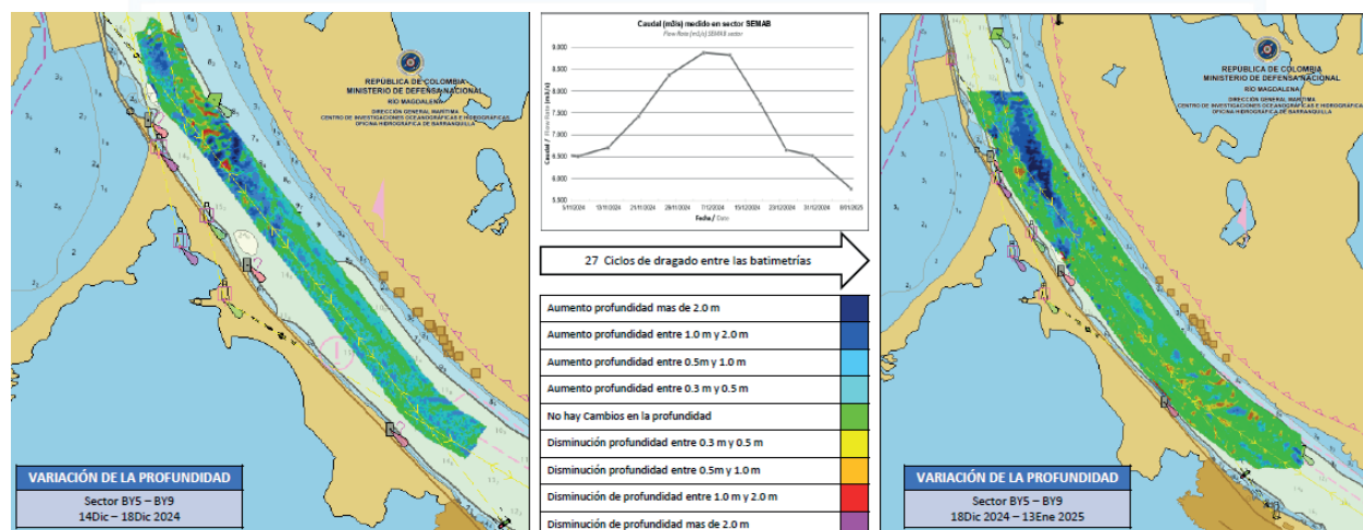
Figura 11. Diferencia de superficie entre el 18 de diciembre y el 13 de enero del 2025.
