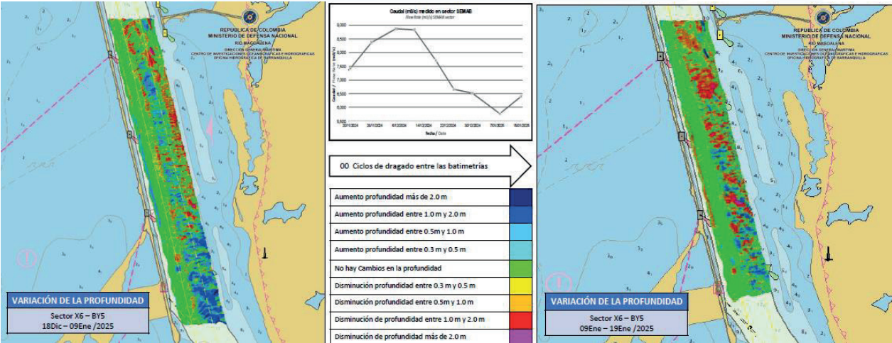
Figura 9. Diferencia de superficie entre el 09 y el 19 de enero del 2025.
