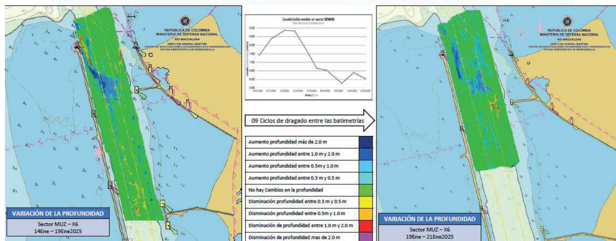
Figura 6. Diferencia de superficie entre el 19 y 21 de enero del 2025.
