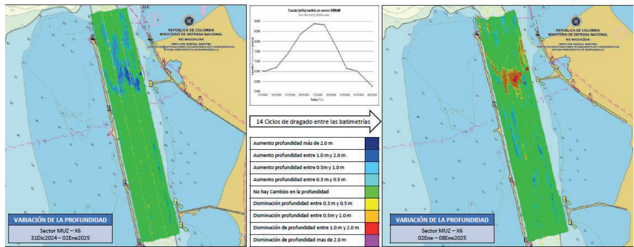
Figura 2. Diferencia de superficie entre el 02 y el 08 de enero del 2025.
