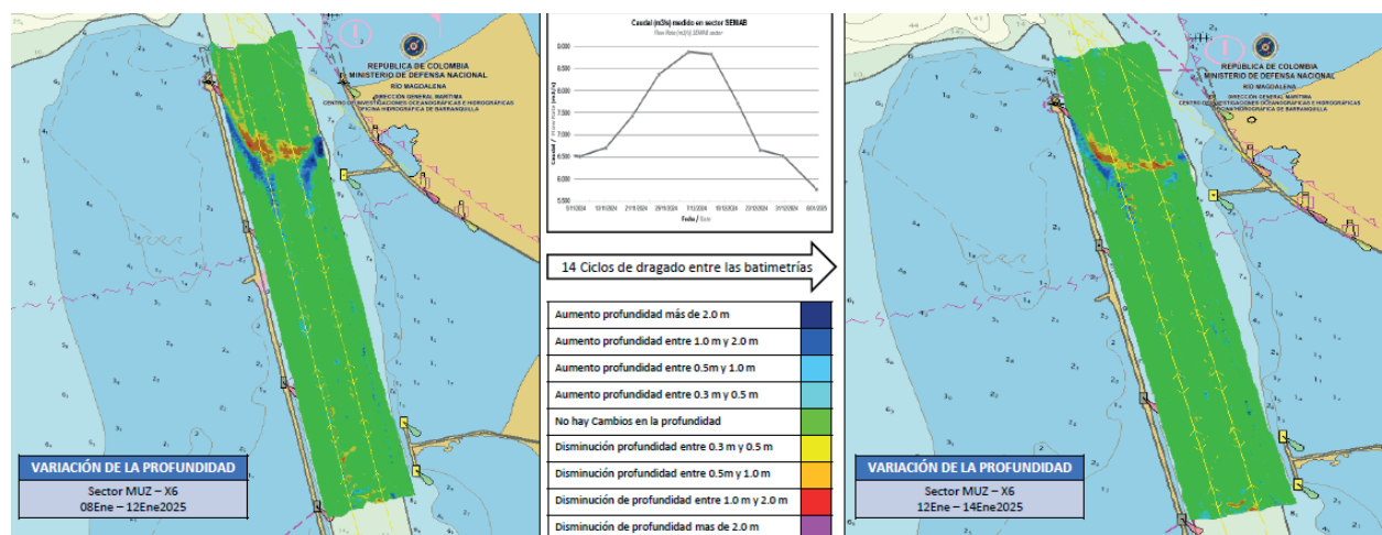
Figura 4. Diferencia de superficie entre el 12 y 14 de enero del 2025.
