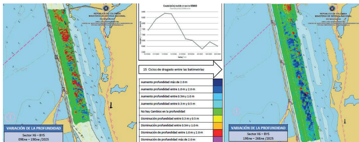
Figura 10. Diferencia de superficie entre el 19 y el 26 de enero del 2025.
