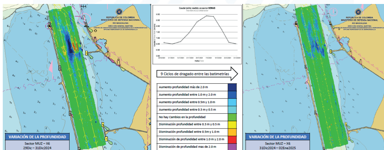
Figura 17. Diferencia de superficie entre el 31 de diciembre y de 02 enero del 2025.
