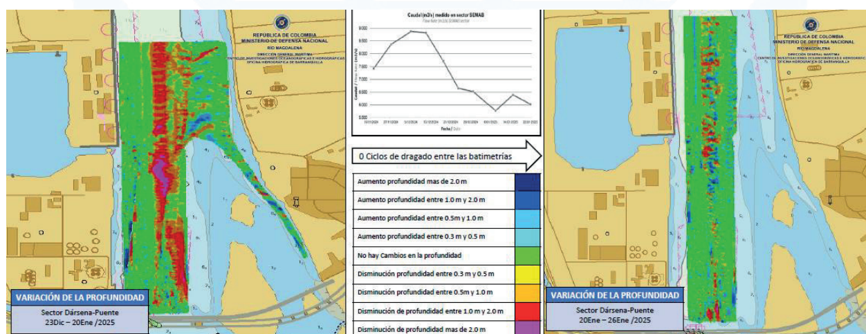
Figura 24. Diferencia de superficie entre el 20 y el 26 de enero del 2025.
