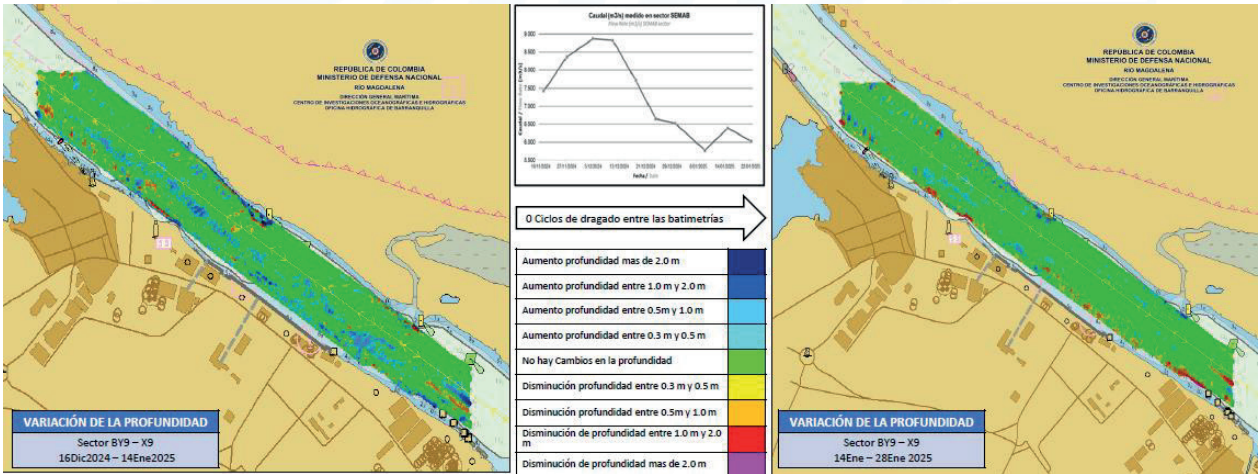
Figura 14. Diferencia de superficie entre el 14 y el 28 de enero del 2025.
