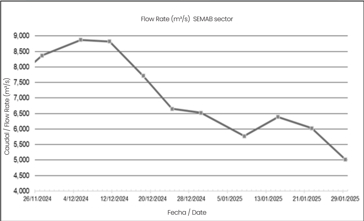
Figura 25. Evolución comportamiento caudal sección transversal km 8+500.
