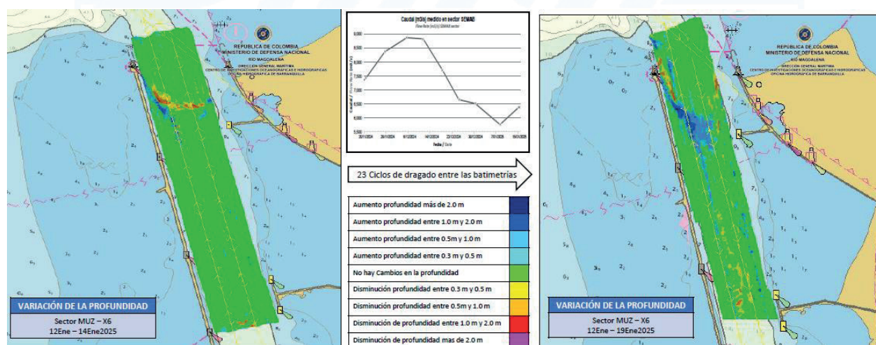
Figura 5. Diferencia de superficie entre el 14 y 19 de enero del 2025.
