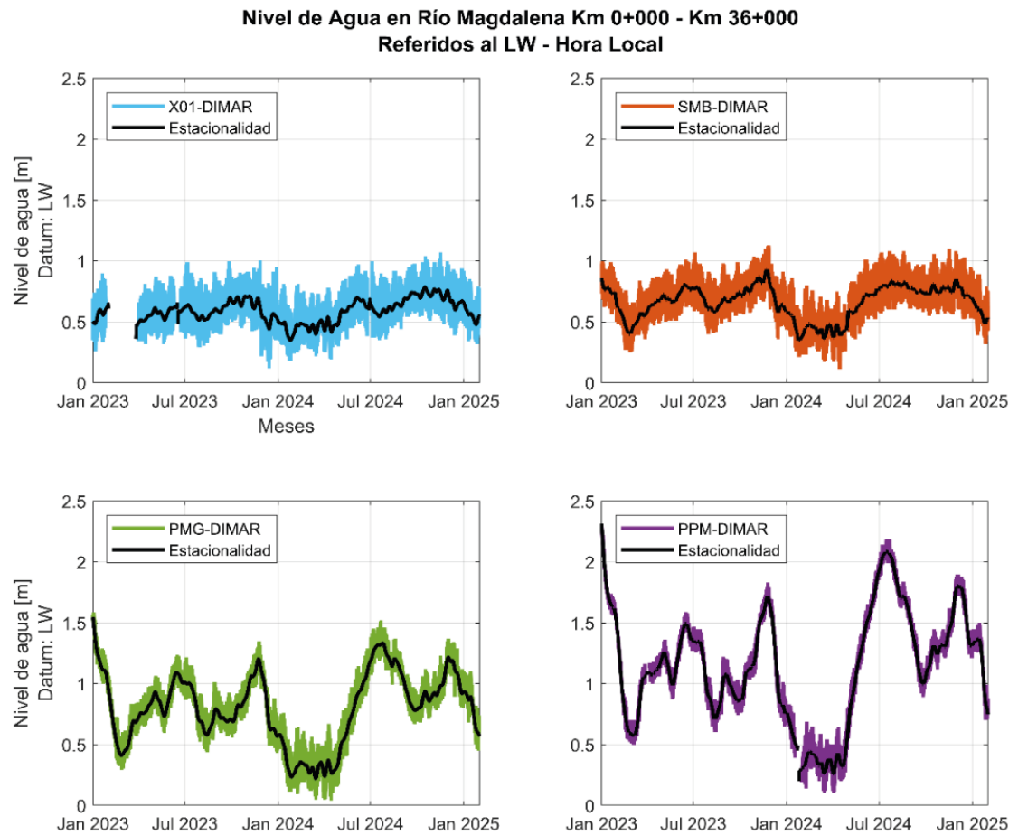
Figura 26. Serie temporal comportamiento niveles de agua y estacionalidad en el Río Magdalena (km 0 al km 36).
