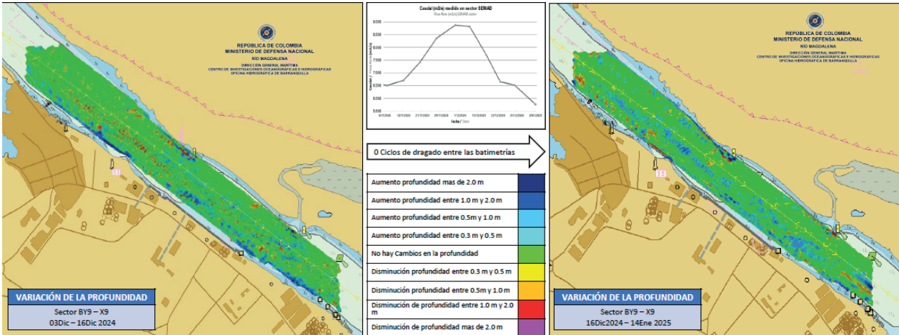
Figura 13. Diferencia de superficie entre el 16 de diciembre y el 14 de enero del 2025.
