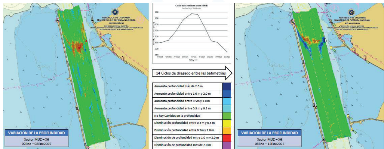
Figura 3. Diferencia de superficie entre el 08 y 12 de enero del 2025.
