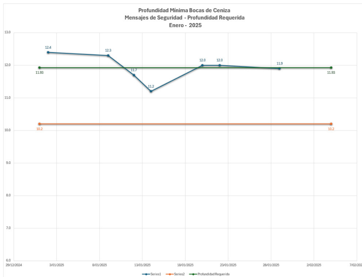
Figura 27. Correlación de profundidad mínima Vs los mensajes de seguridad durante el mes enero a enero del 2025.
