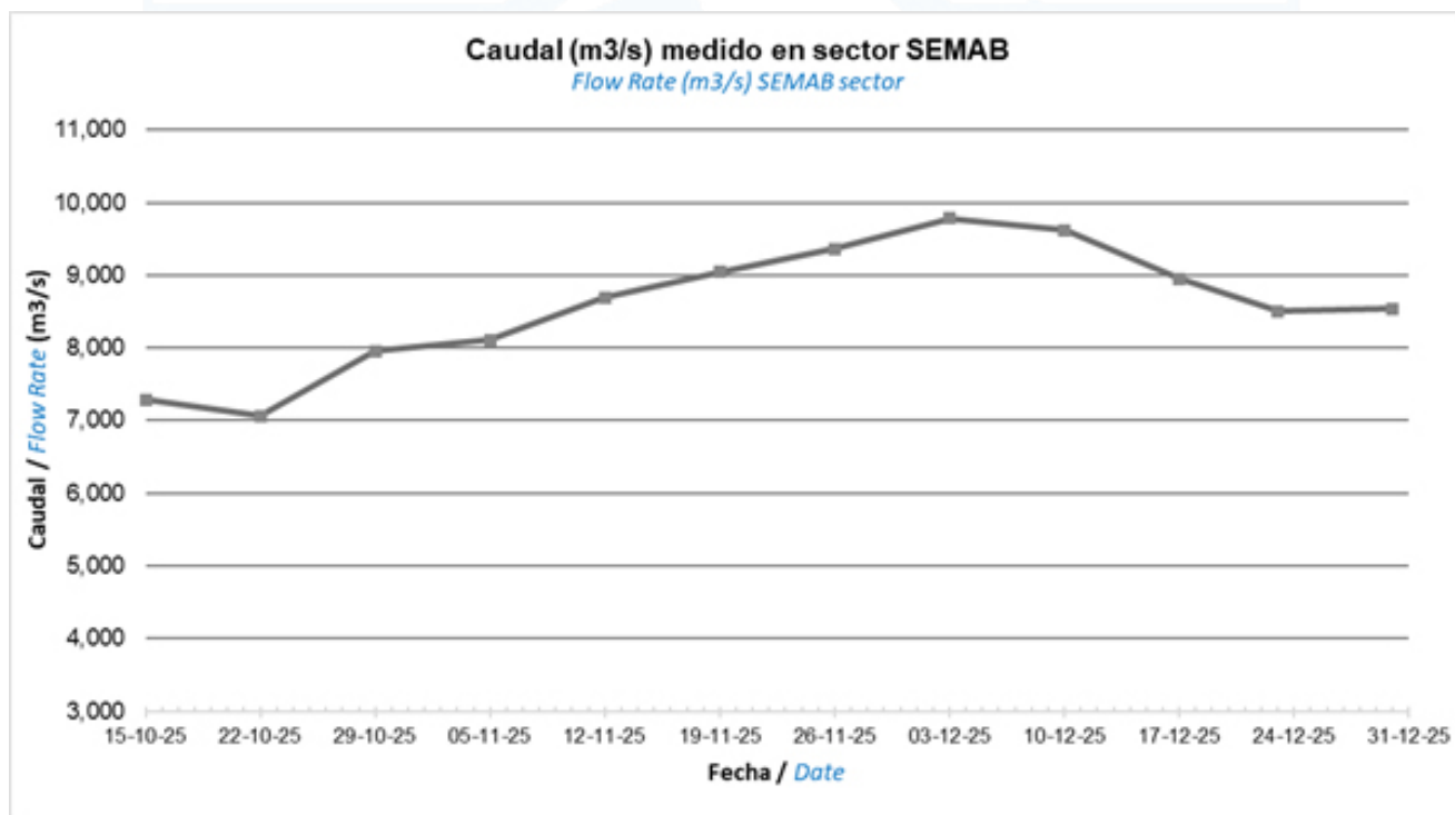
Figura 49. Evolución comportamiento caudal sección transversal km 8+500.
