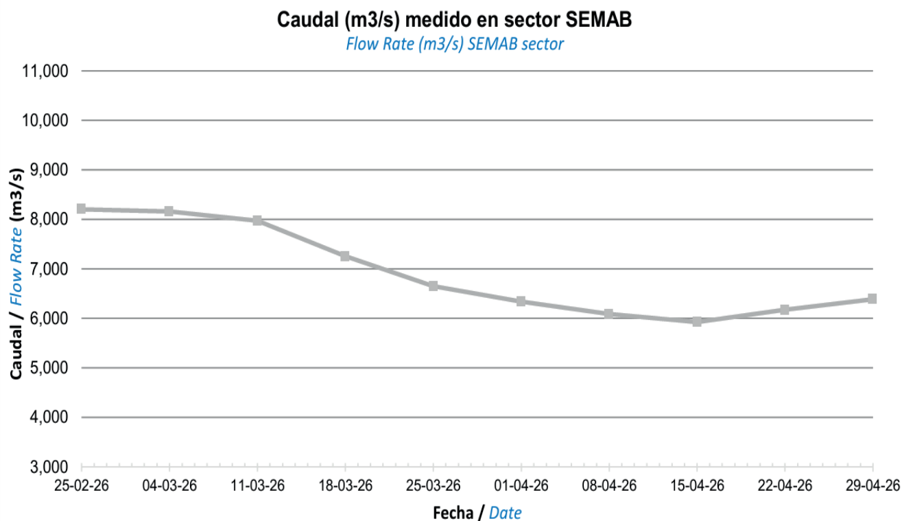
Figura 34. Evolución comportamiento caudal sección transversal km 8+500.
