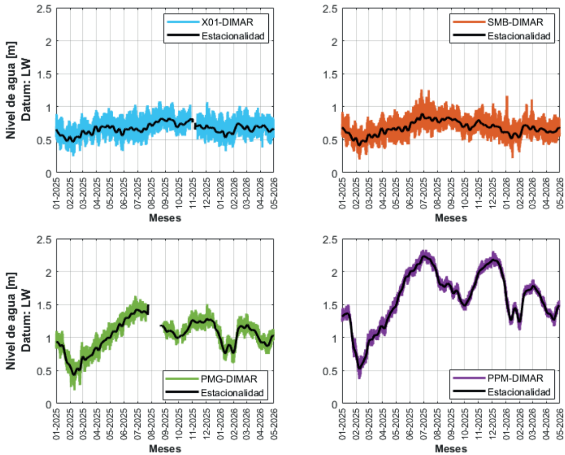
Figura 35. Serie temporal comportamiento niveles de agua y estacionalidad en el Río Magdalena (km 0 al km 36).
